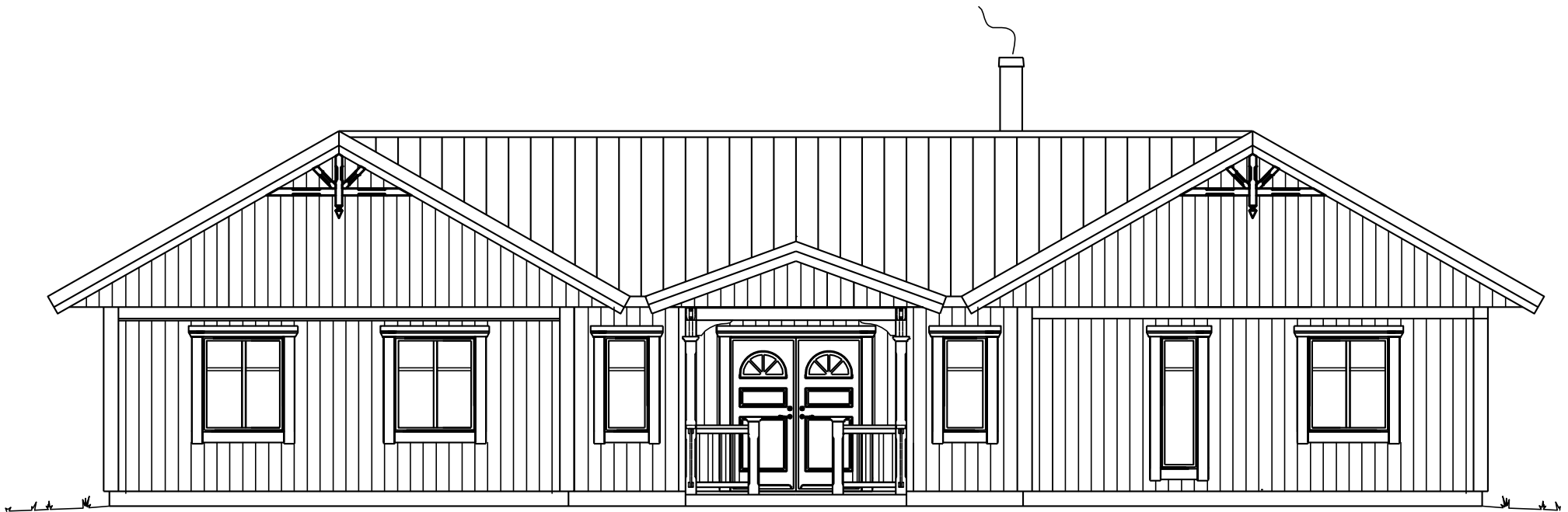
ENTRÉFASAD
